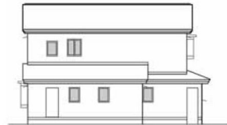
■北立面図
