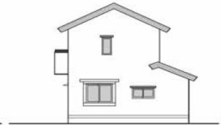
■東立面図
