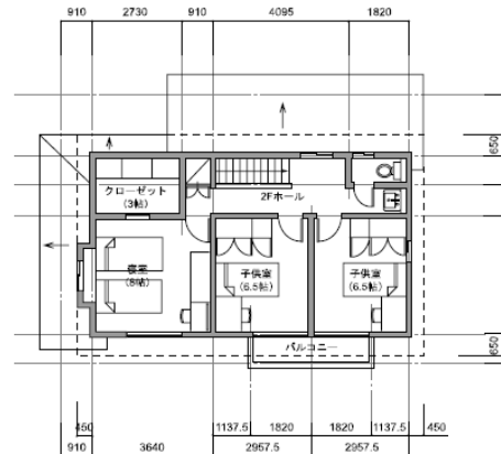
■2階平面図
