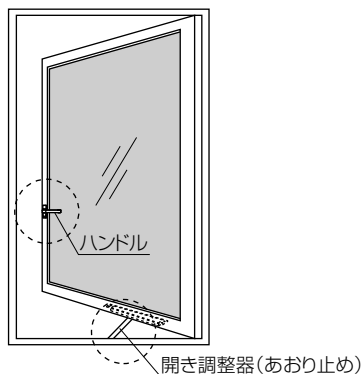
(MTG-70 MTG-70高性能サッシ)
