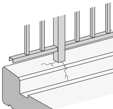
⑫ 手すりの建物取り付け部に、コンクリートのひび割れがある。
