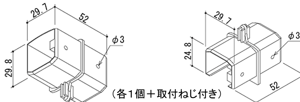
連結材(上・下) FIN-J
